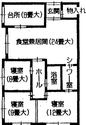
米軍家族住宅の間取り (120㎡)
